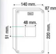
BMBOX -2P 2 POLE
