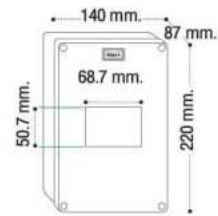
BMBOX -3P 3 POLE
