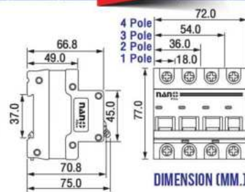
4 Pole 1000VDC
