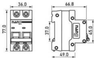
2 Pole 10 kA
