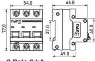
3 Pole 6 kA
