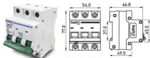
3 Pole 6 kA
