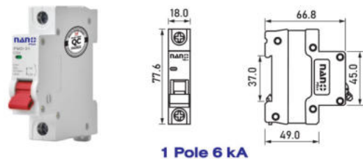
1 Pole 6 kA
