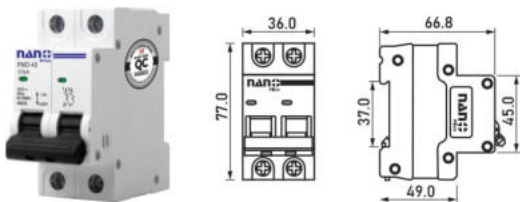
2 Pole 10 kA
