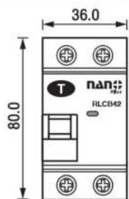
2 Pole 10 kA
