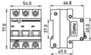
3 Pole 6 kA
