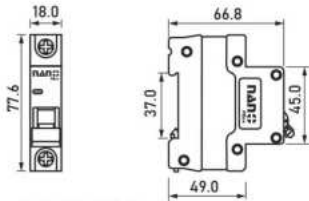
1 Pole 6 kA
