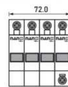
3P+N 10-20 kA
