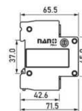
3P+N 10-20 kA
