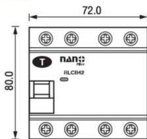
4 Pole 10 kA
