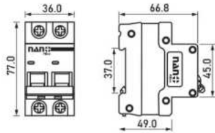
2 Pole 10 kA
