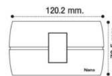
Switch Curve Plate size : 2 module แผงหน้ากากขอบเหลี่ยมโค้ง ขนาด : 2 ช่อง
