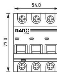
3 Pole 6 kA
