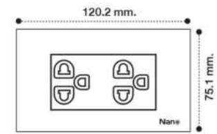
CP55R-W / CP55R-B Duplex 3 Pin Socket ชุด เต้ารับเข็ม มีกราวน์ และปุ่มนิรภัย
