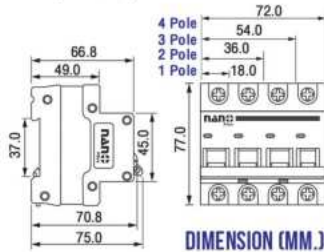
เซอร์กิตเบรกเกอร์ DC (MCB) 1 Pole 6 kA
