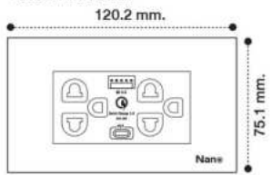
CP-66U-W / CP-66U-B Duplex 3 pin socket 16A ~250VAC +USB Quick Charger (QC 3.0,PD)20W USB Type A+Type C ชุดเต้ารับเข็มมีกราวน์ ปุ่มนิรภัย 16A ~250VAC + เต้ารับชาร์จเร็วควิกชาร์จ 3.0 พดี 20 วัตต์ USB Type A+Type C
