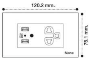
CP05U-W / CP05U-B 3 Pin Socket 16A ~250VAC with safety shutter and Dual USB Charger 2.1A~5VDC ชุด เต้ารับเข็ม มีกราวน์ และปุ่มนิรภัย + USB 2.1 แอมป์ 5 บาร์
