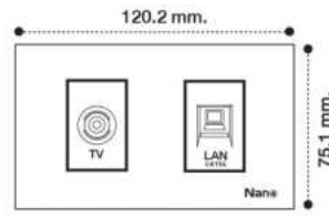
CP-TVPC-W / CP-TVPC-B TV Socket (DIN TYPE) and LAN Socket (CAT5E) ชุด เต้ารับทีวี + เต้ารับคอมพิวเตอร์ CAT5E
