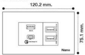
CP-3A1C-W / CP-3A1C-B Dual USB Quick Charger(QC 3.0,PD) 20W USB Type A+Type C +USB Charger 2.1A~5VDC Type A(2 Port) ชุดเต้ารับชาร์จเร็วควิกชาร์จ 3.0 และพดี 20 วัตต์ USB Type A+Type C + เต้ารับ USB 2.1 แอมป์ 5 บาร์ Type A (2 ช่อง)
