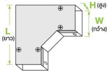
เปิดบน HORIZONTAL ELBOW
