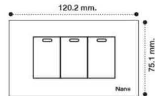
CP111-W / CP111-B 1 Way Switch with Luminous x 3 pcs. ชุดสวิตช์ 1 ทาง แบบมีพรายน้ำ x 3 ตัว
