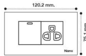
CP15-W / CP15-B 3 Pin Socket +1 Way Switch with Luminous ชุด เต้ารับเข็ม มีกราวน์ และปุ่มนิรภัย + สวิตช์ 1 ทางแบบมีพรายน้ำ
