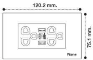
CP55U-W / CP55U-B Duplex 3 pin socket 16A ~250VAC with safety shutter and Dual USB Fast charger 3.1A~5VDC ชุดเต้ารับเข็มมีกราวน์ ปุ่มนิรภัย + USB 3.1 แอมป์ 5 บาร์ 2 ช่อง
