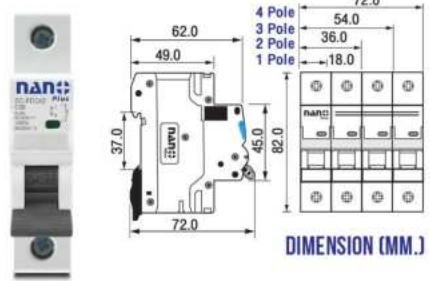
เซอร์กิตเบรกเกอร์ DC (MCB) 1 Pole 10 kA
