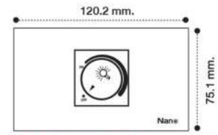
CP-DM-W / CP-DM-B Dimmer Module 300W ~250VAC ชุด สวิตช์หรี่ไฟ 300 วัตต์ 250 โวลต์
