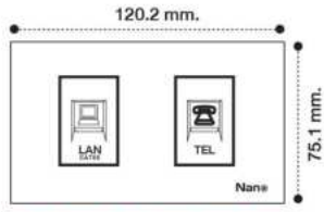
CP-PCTEL-W / CP-PCTEL-B Telephone socket (6P4C) + LAN Socket (CAT5E) ชุด เต้ารับโทรศัพท์ + เต้ารับคอมพิวเตอร์ CAT5E
